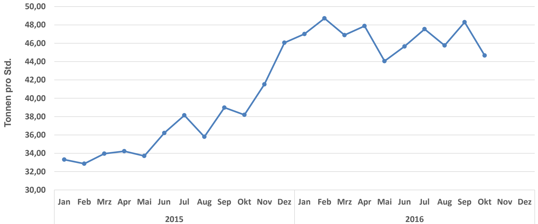
Leistung in Tonnen/Maschinenstunde
